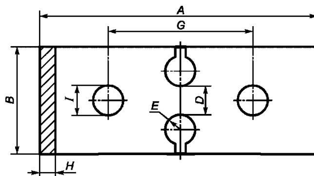
Рисунок 3 - Испытуемый образец, тип 2
