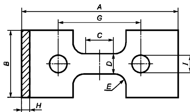
Рисунок 4 - Испытуемый образец, тип 3
