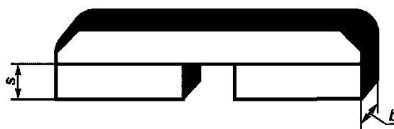
Образец, выполненный нагретым инструментом в раструб
