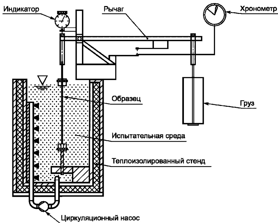
Рисунок 5 - Стенд для испытаний на ползучесть при растяжении
