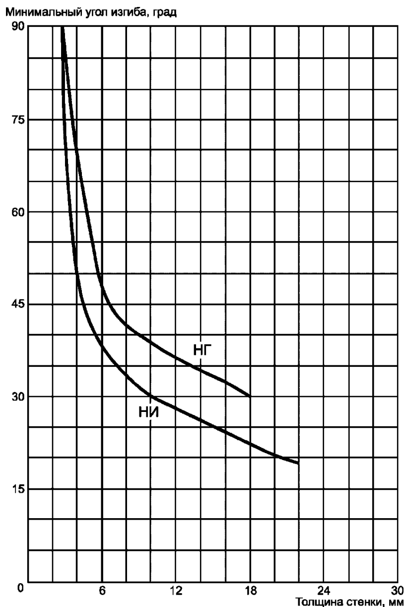
Рисунок В.4 - Минимальный угол изгиба для ПВХФ в зависимости от толщины для разных методов сварки (нижняя кривая - для сварки нагретым инструментом встык, верхняя - для прутковой сварки нагретым газом)
