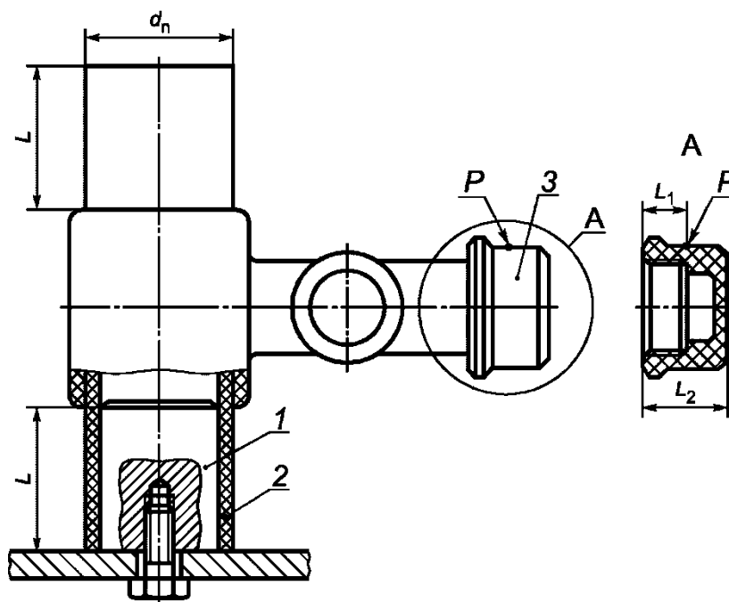
1 - стальной сердечник; 2 - труба; 3 - крышка отвода; L = d_e ; L_1 = L_2/2 ; P - место нанесения удара
