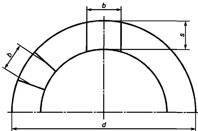
Рисунок 11 - Способы вырезания образцов из трубы
