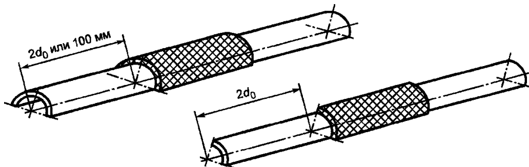
Рисунок 15 - Подготовка испытываемых образцов
