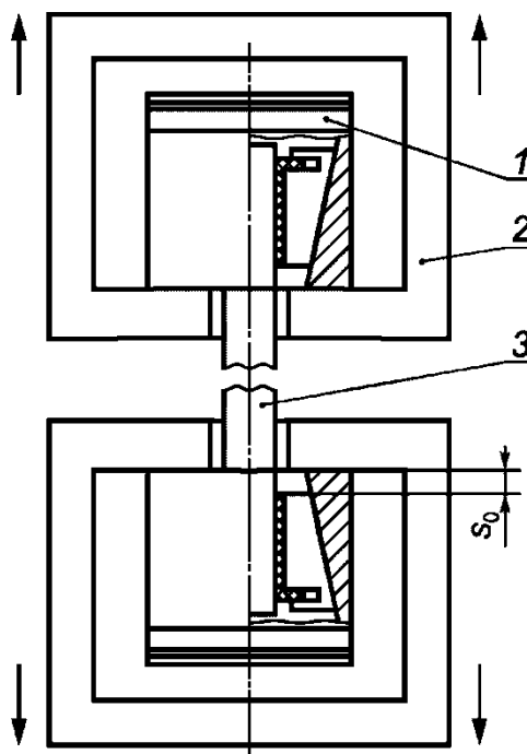
1 - зажим; 2 - приспособление для испытания; 3 - образец
